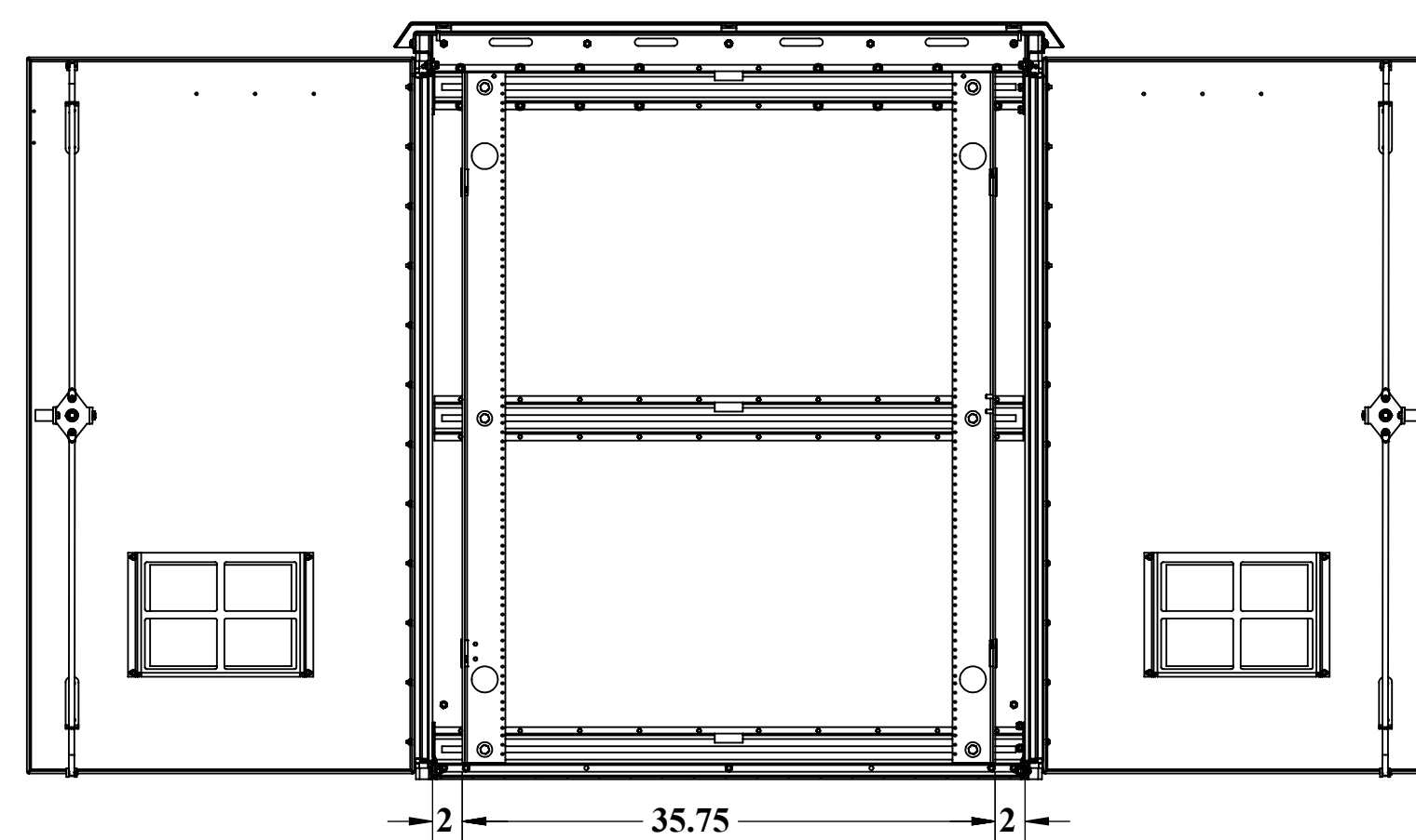
SECTION A-A SCALE 1 : 12
