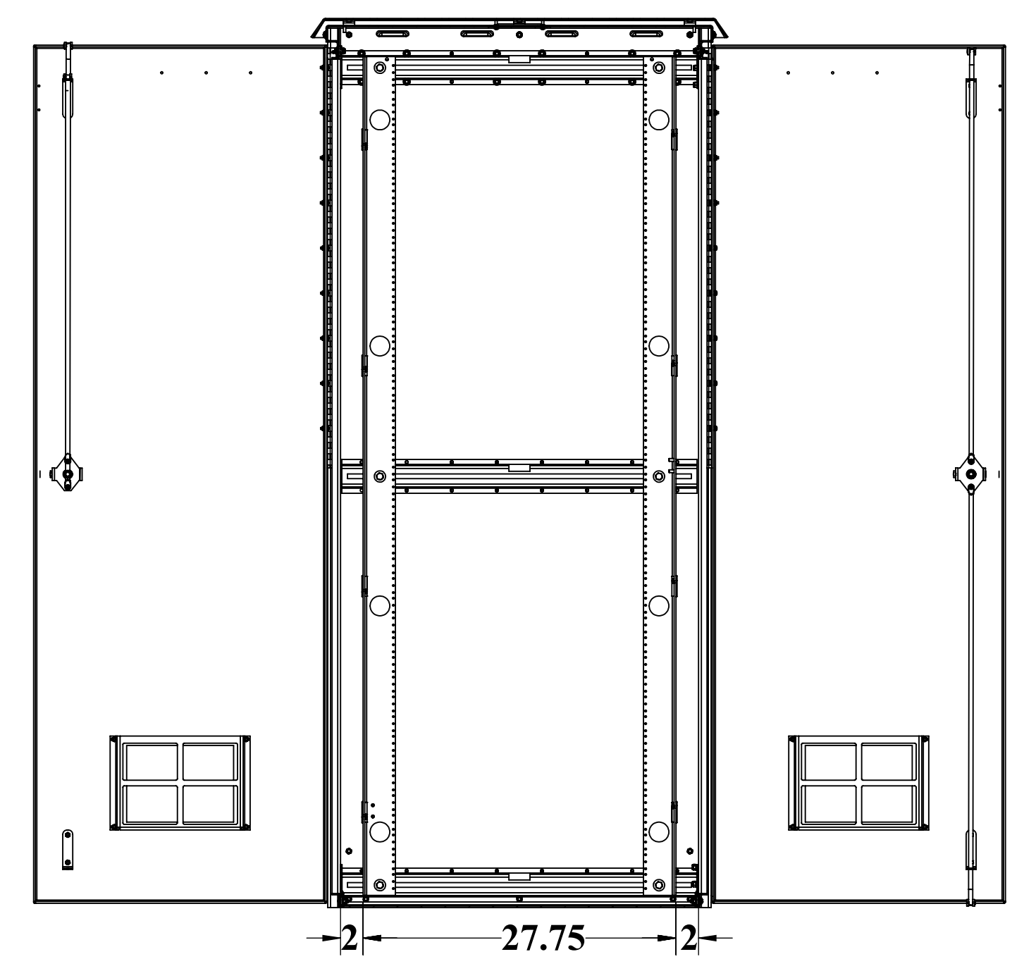
SECTION A-A SCALE 1:12
