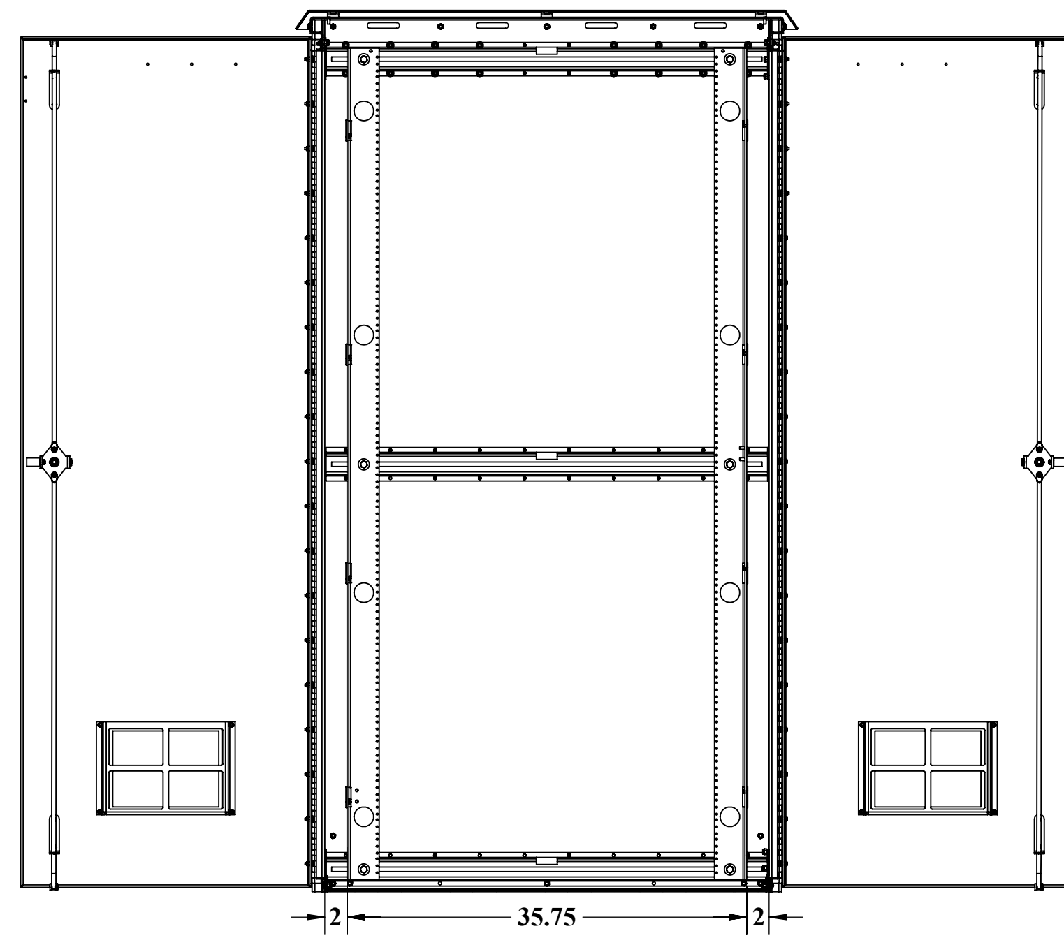
SECTION A-A SCALE 1 : 12
