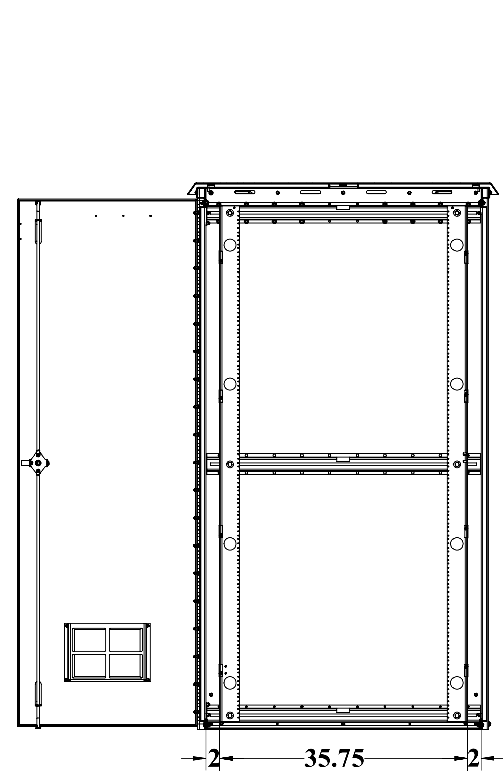
SECTION A-A SCALE 1:14
