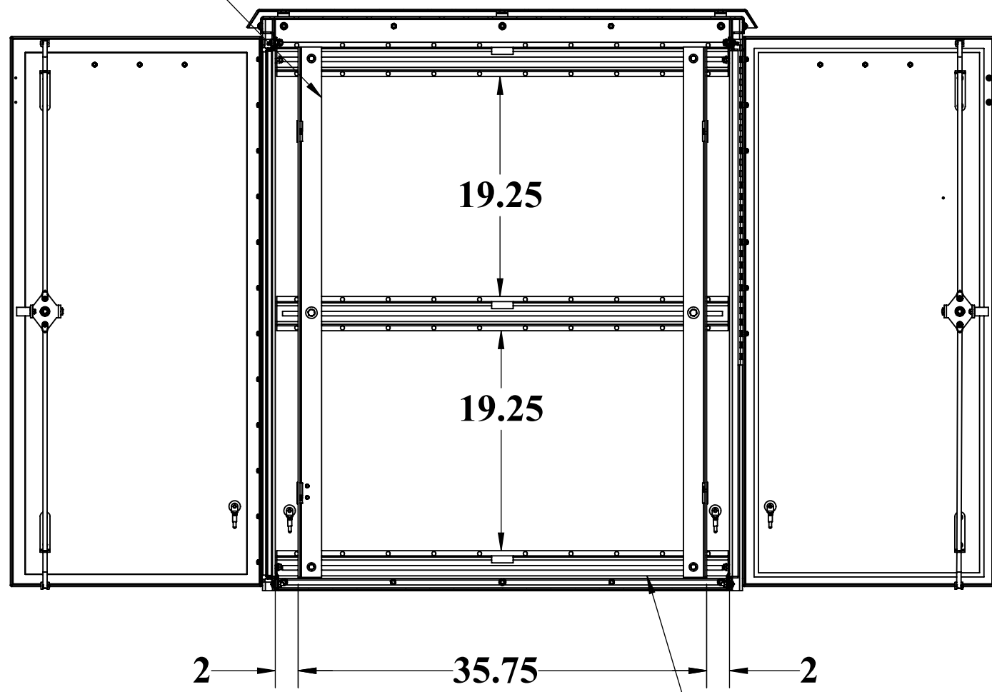
SECTION A-A
