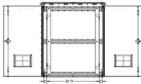
SECTION A-A SCALE 1 : 12
