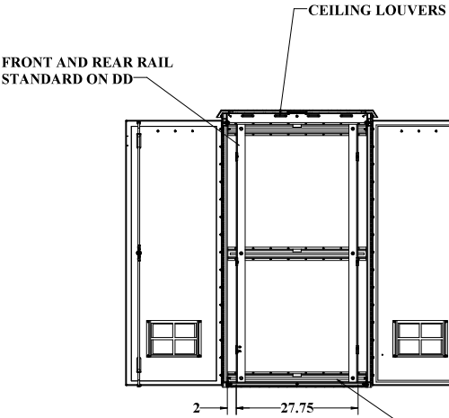
SECTION A-A SCALE 1 : 12
